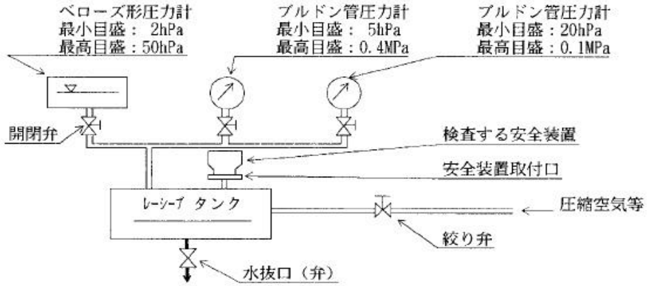
例1 最高試験圧力1MPaの試験装置
