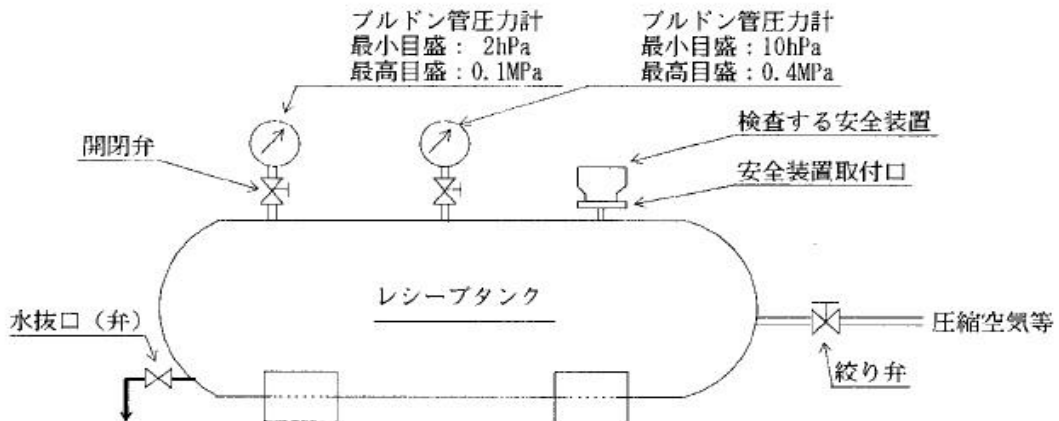
例2 最高試験圧力0.4MPaの試験装置
