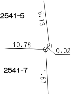
拡大図 縮尺 1:200
