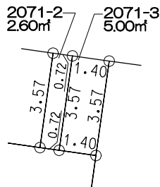
拡大図 縮尺 1:200
