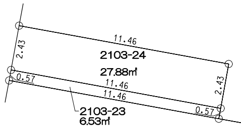
拡大図 縮尺 1:200
