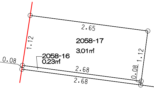
拡大図 縮尺 1:50
