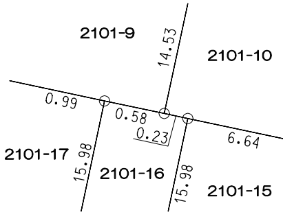
拡大図 縮尺 1:50
