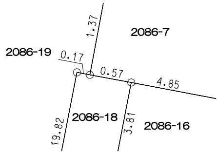
拡大図 縮尺 1:50
