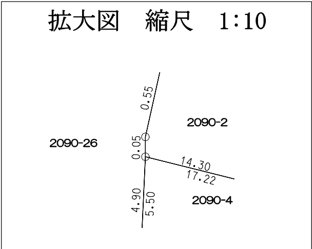
拡大図 縮尺 1:10
