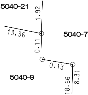
拡大図 縮尺 1:10
