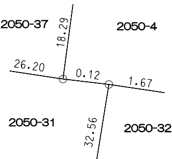
拡大図 縮尺 1:10
