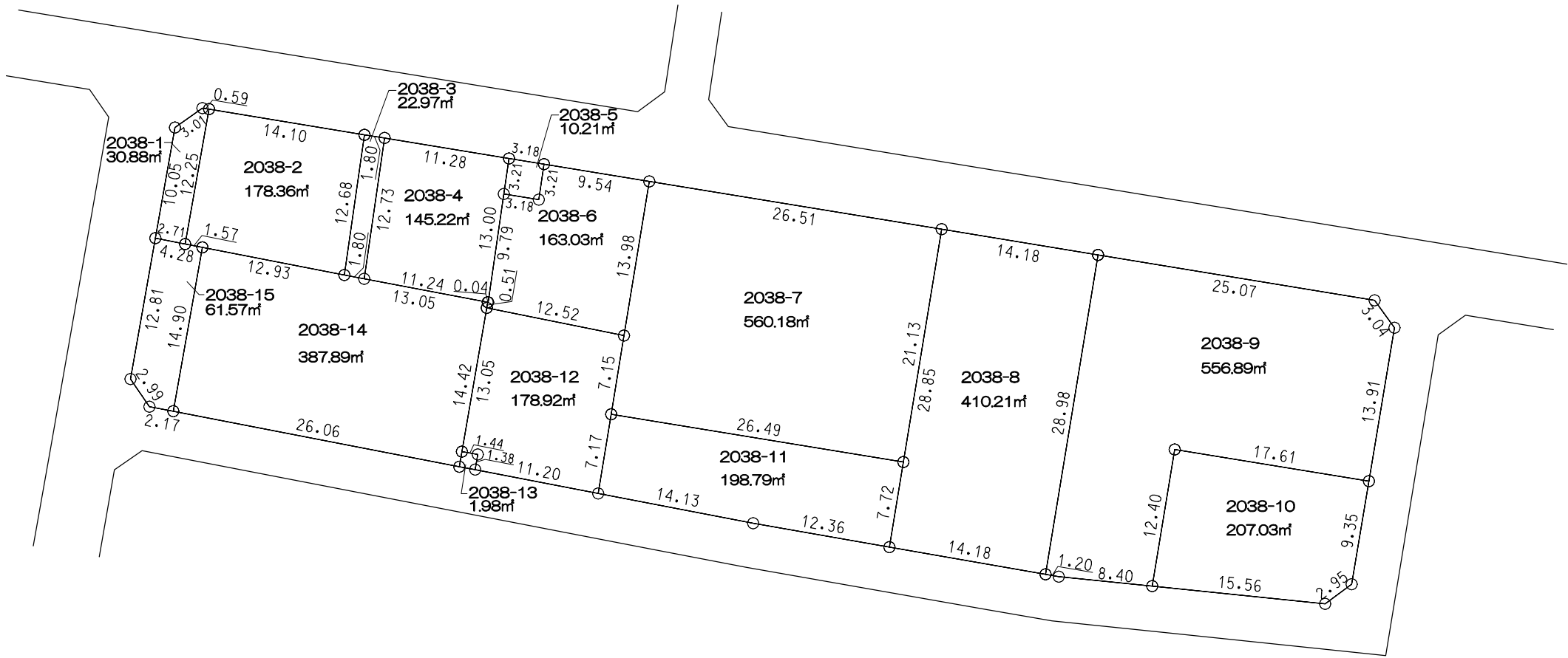
拡大図 縮尺 1:10
