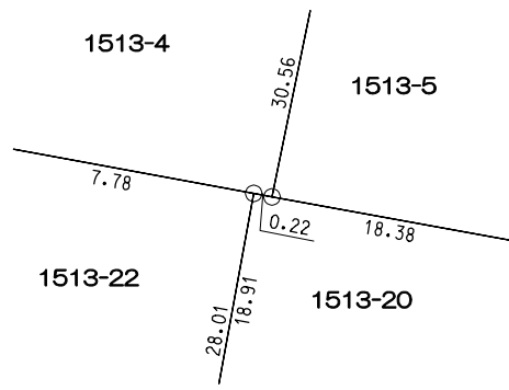
拡大図 縮尺 1:100
