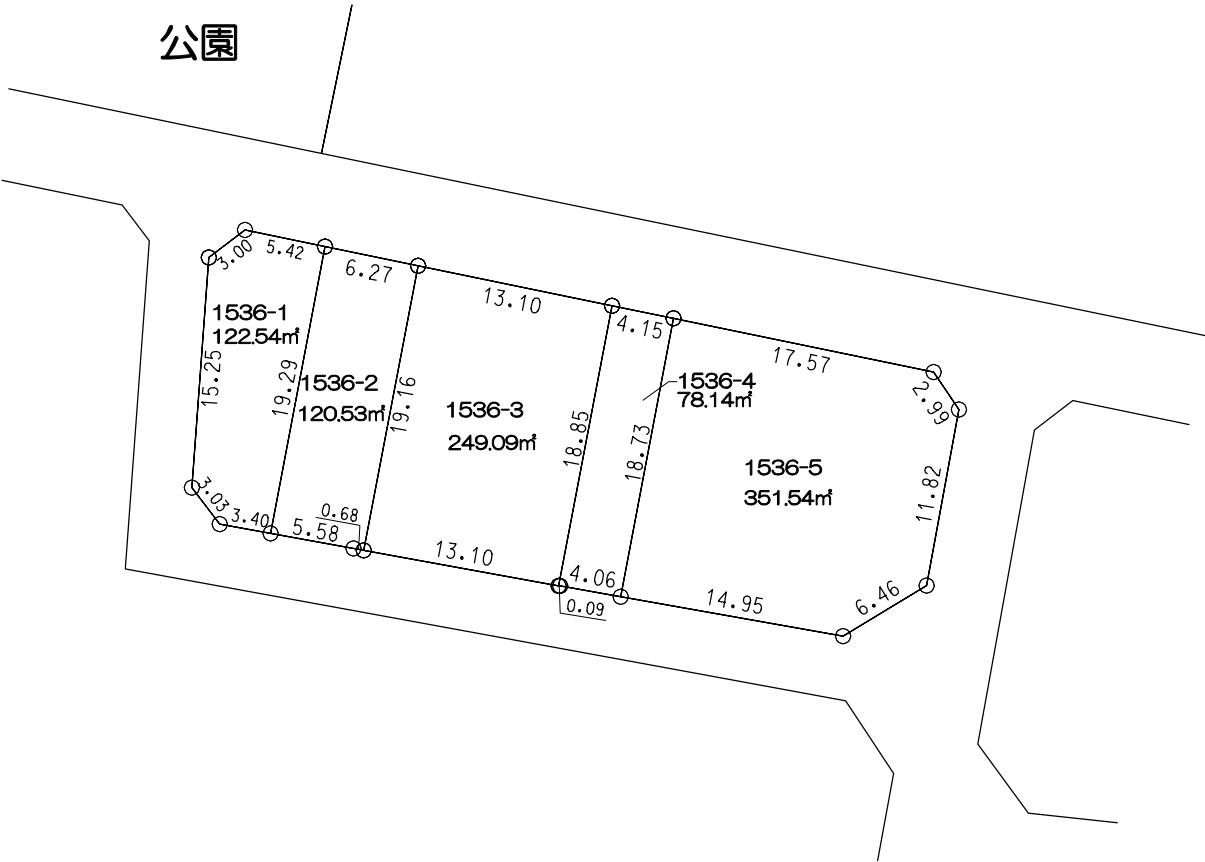
拡大図 縮尺 1:10
