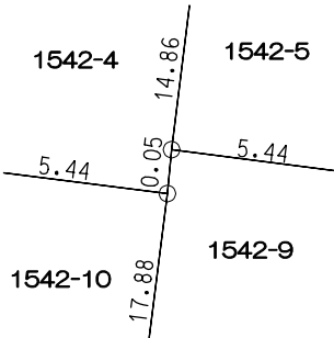
拡大図 縮尺 1:10
