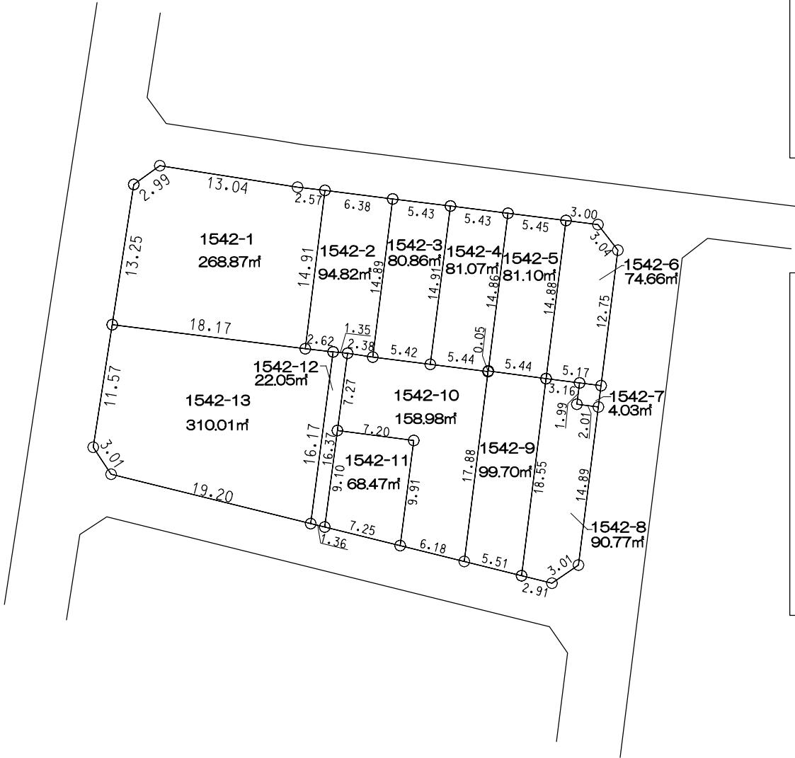
拡大図 縮尺 1:200
