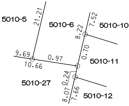
拡大図 縮尺 1:50
