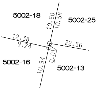
拡大図 縮尺 1:10
