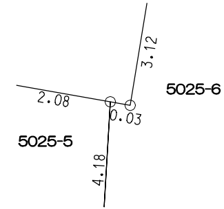
拡大図 縮尺 1:10
