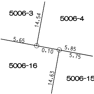
拡大図 縮尺 1:10
