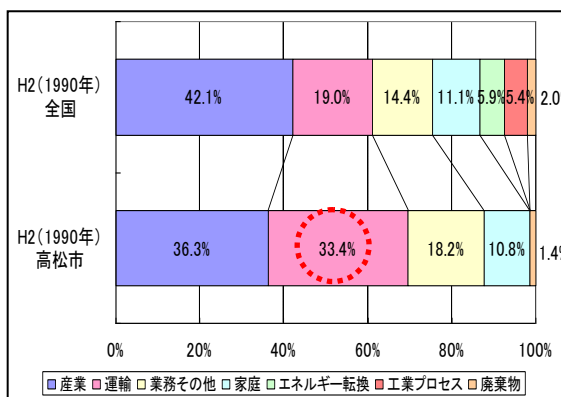
図 2.46 部門別CO 2 排出量
