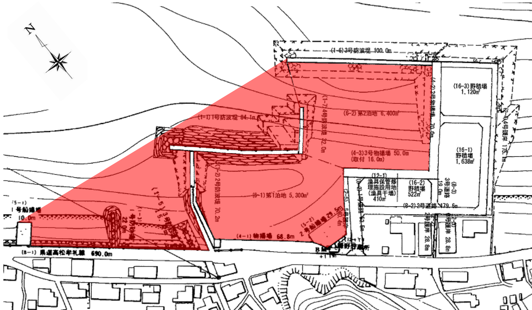
泊地区分平面図（鎌野漁港）
