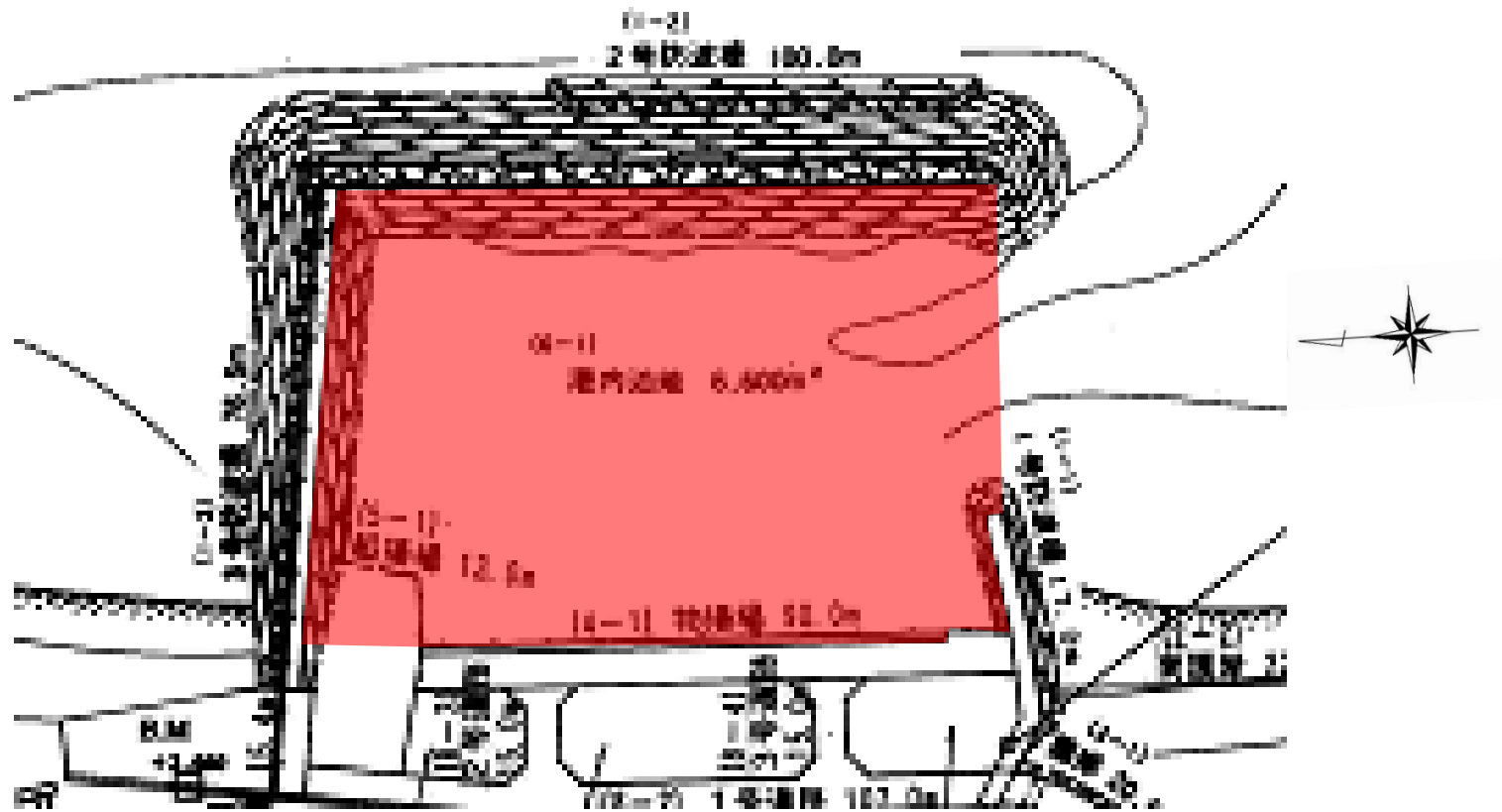
泊地区分平面図（篠尾漁港）
