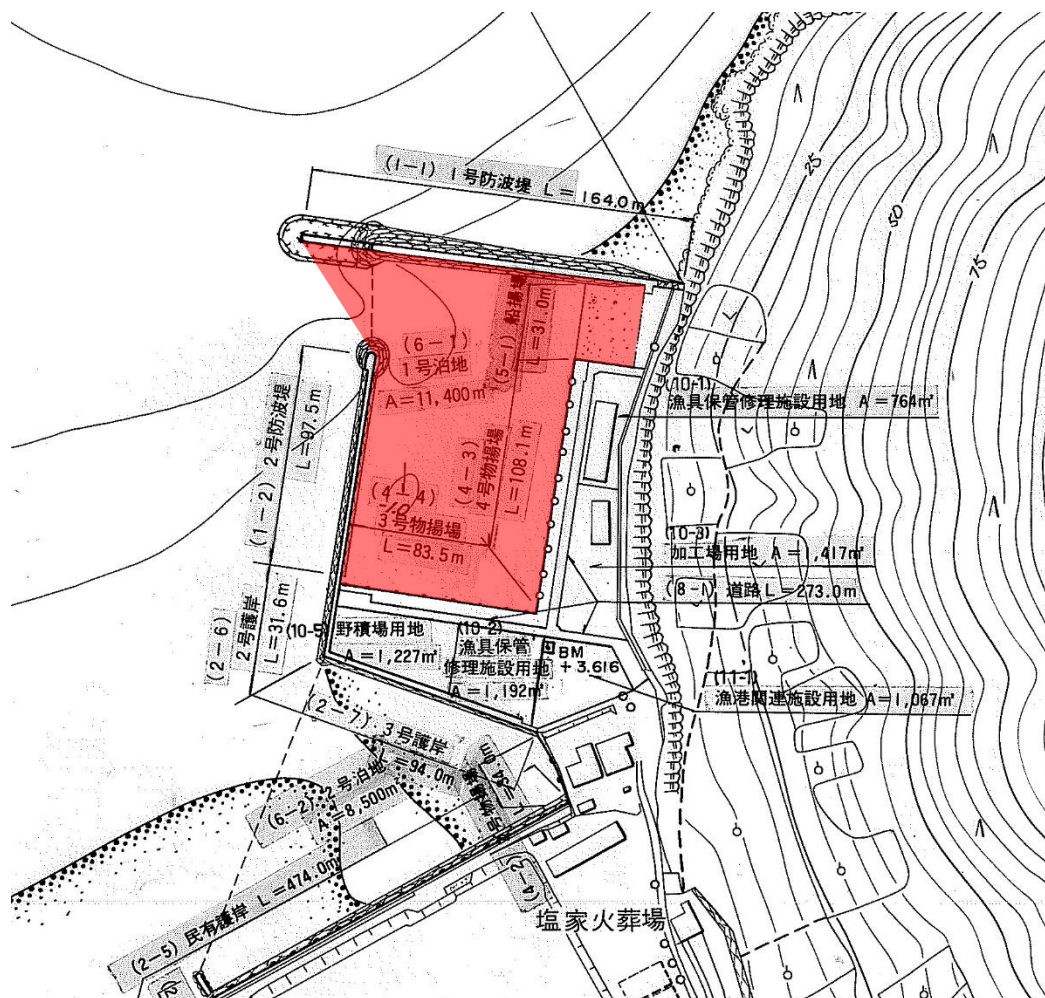
泊地区分平面図（亀水漁港）
