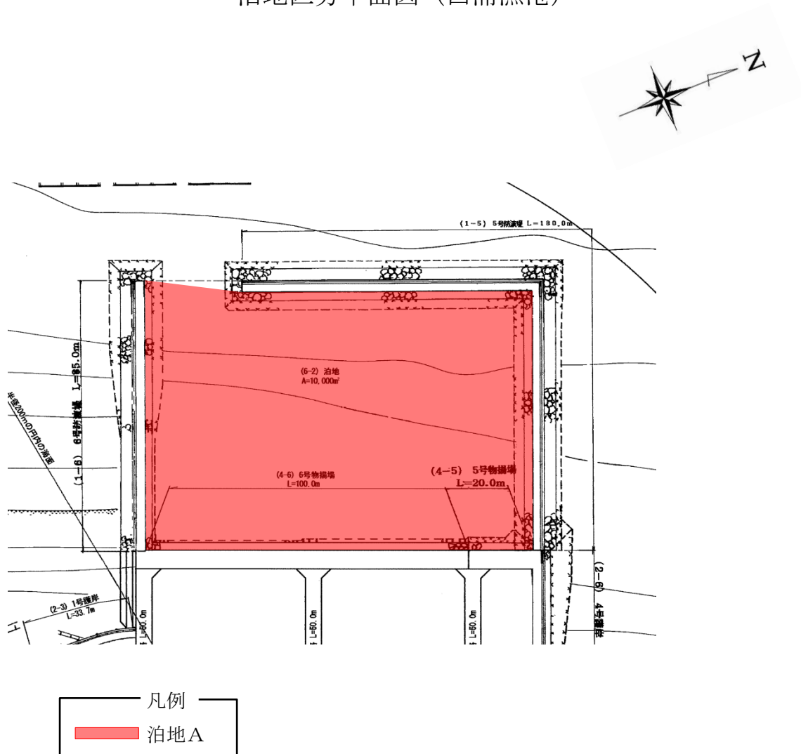
泊地区分平面图（西浦漁港）
