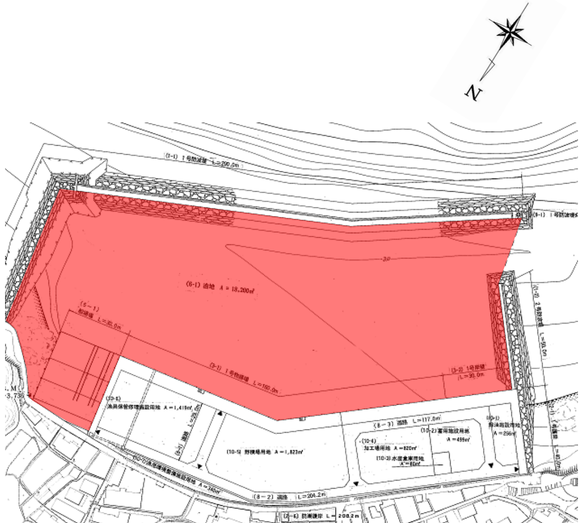
泊地区分平面图（男木漁港）
