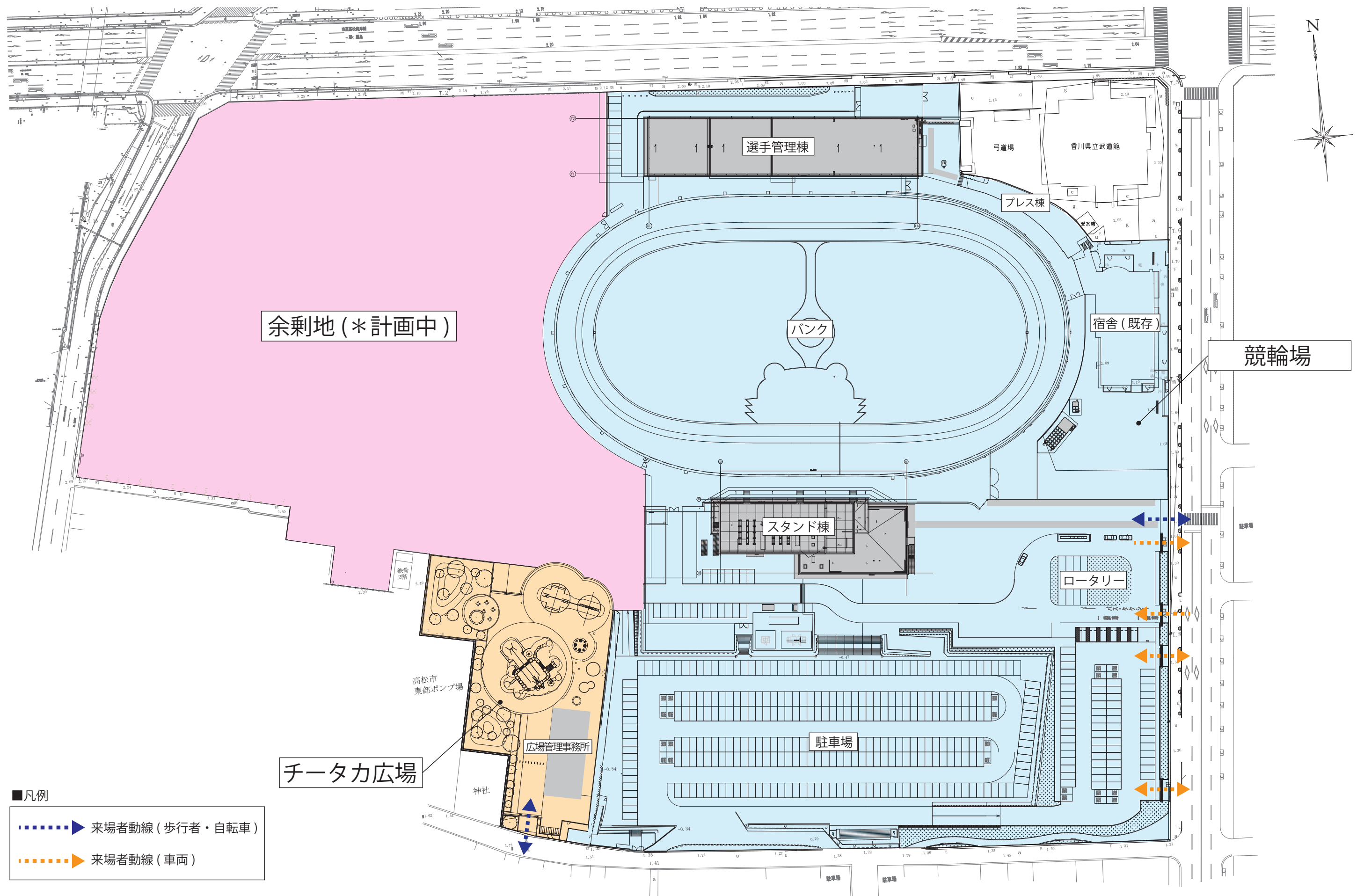
高松競輪場再整備事業 計画図
