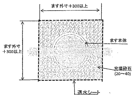
平面図
