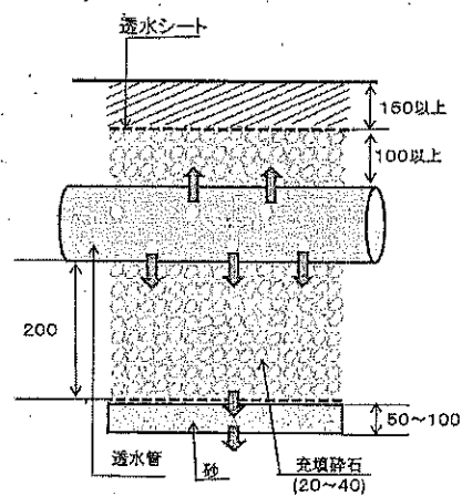
横断面図
