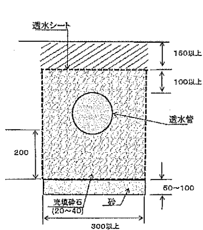
縦断面図
