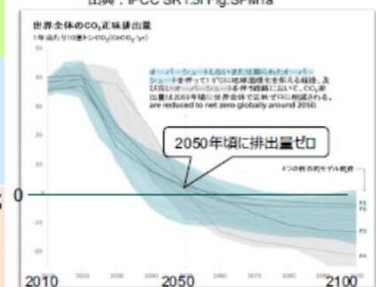
図：1.5℃経路における世界全体のCO 2 排出量 出典：IPCC SR1.5I Fig. SPM3a
