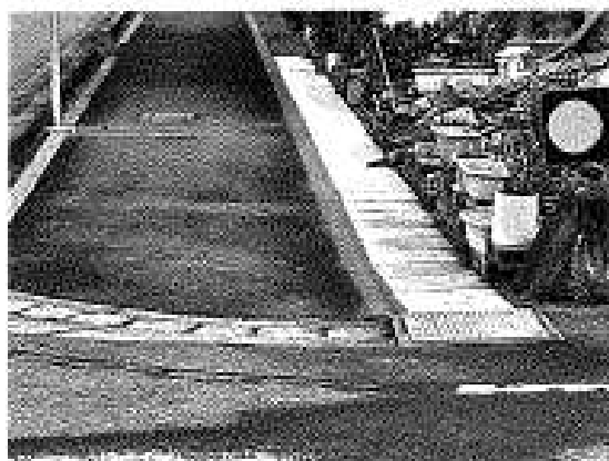
県道側溝蓋設置（香川町）
