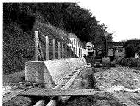
急傾斜工事（西谷地区）
