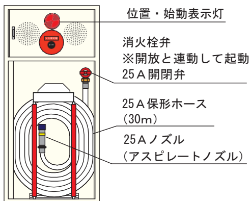
(広範囲型2号消火栓の構成例)
