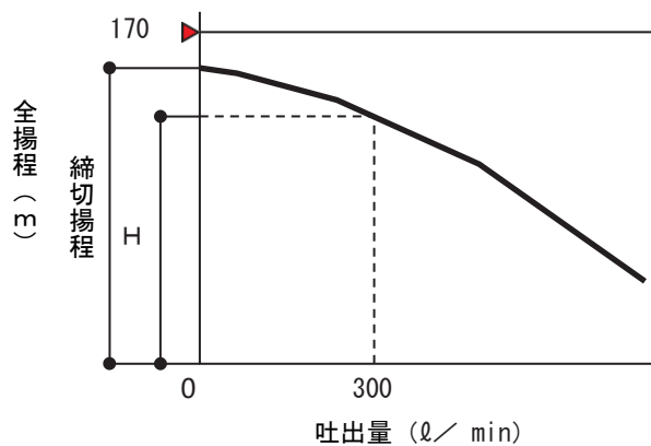
〔ポンプ揚程曲線図〕
