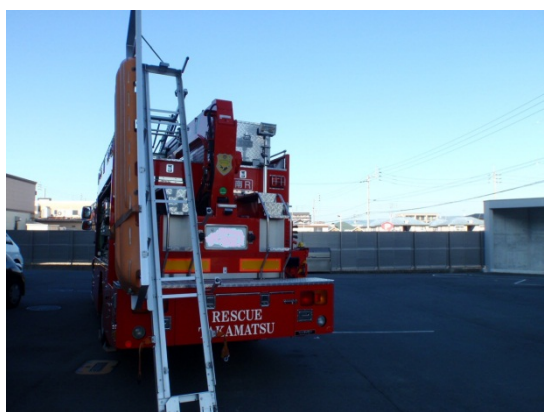
車両後方より三連梯子降下状況
