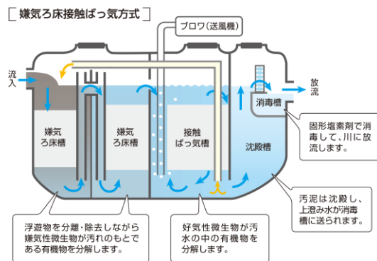
合併処理浄化槽の構造
