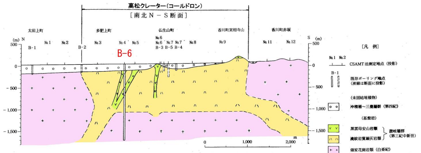
図10「高松クレーターの地下構造（長谷川、2007）」
