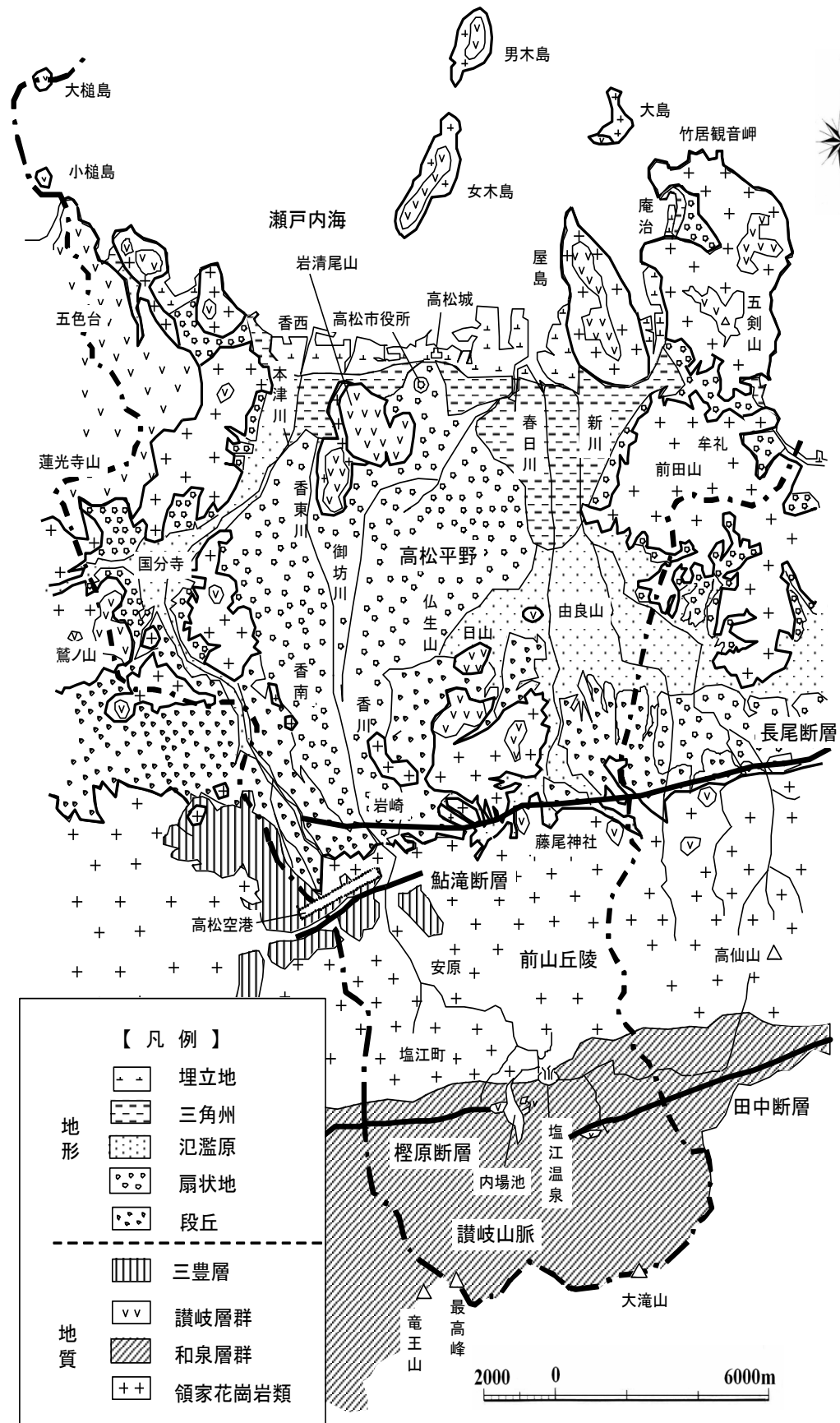
図12 「高松市の地形と地質」 (長谷川修一原図)
