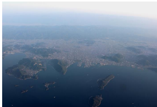
図4 瀬戸内海から高松平野の地形
