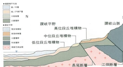
図9 「讃岐平野の地下構造模式図」
