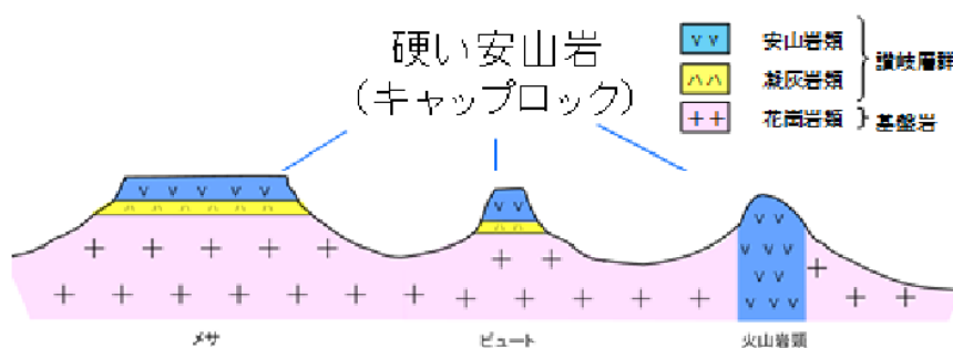
図2 讃岐平野の残丘の地形と地質
