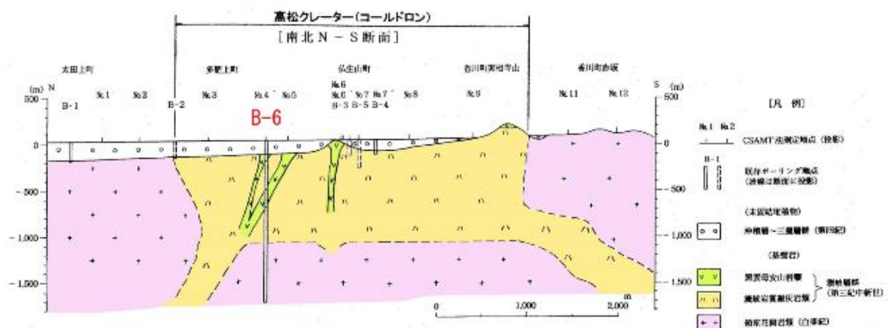
図「高松クレーターの地下構造(長谷川、2007)」
