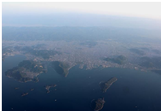
図3 瀬戸内海から高松平野の地形
