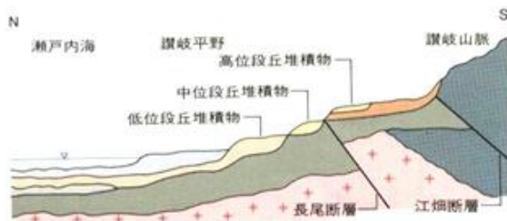
図8 「讃岐平野の地下構造模式図」
