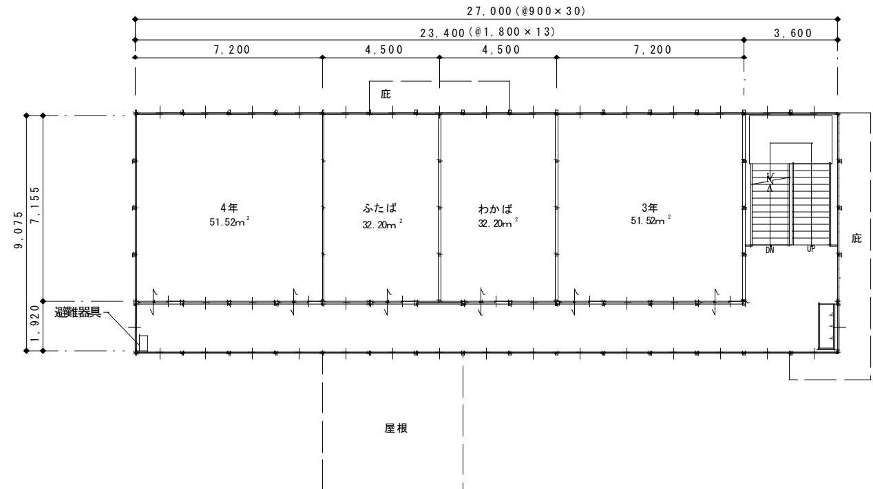
2 階平面図 1/100
