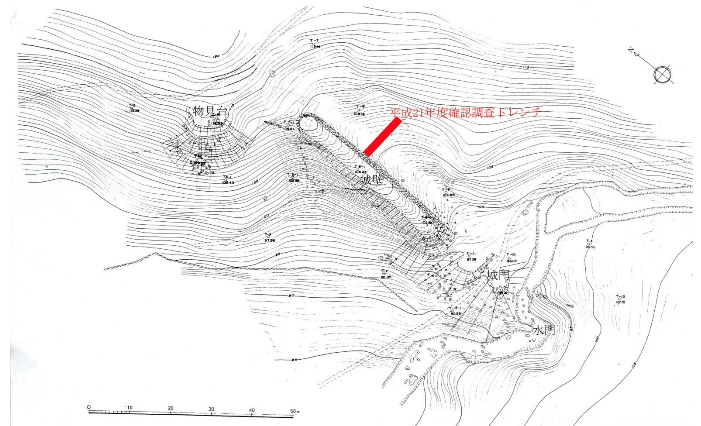
(浦生石塁測量図一遺構配置と平成21年度調査地点一)
