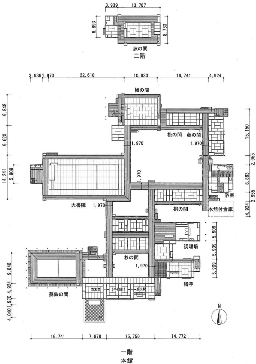
披雲閣（旧松平家高松別邸）平面図
