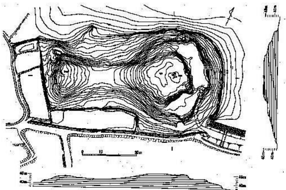
三谷石舟古墳実測図
