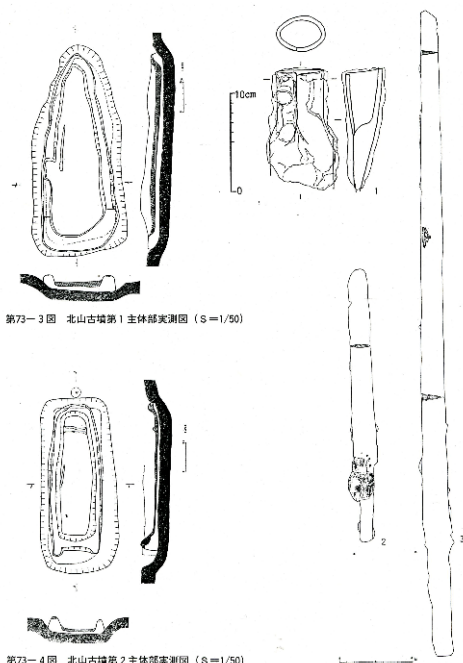
第73-4図 北山古墳第2主体部実測図 (S=1/50)
