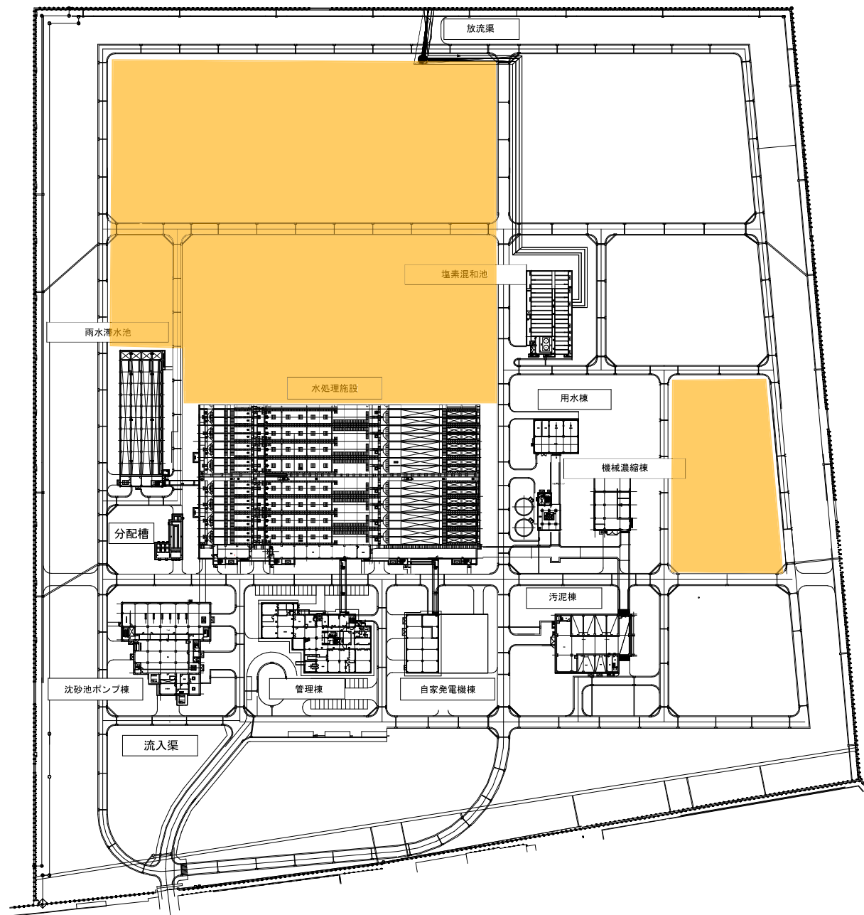
香東川浄化センター 平面図
