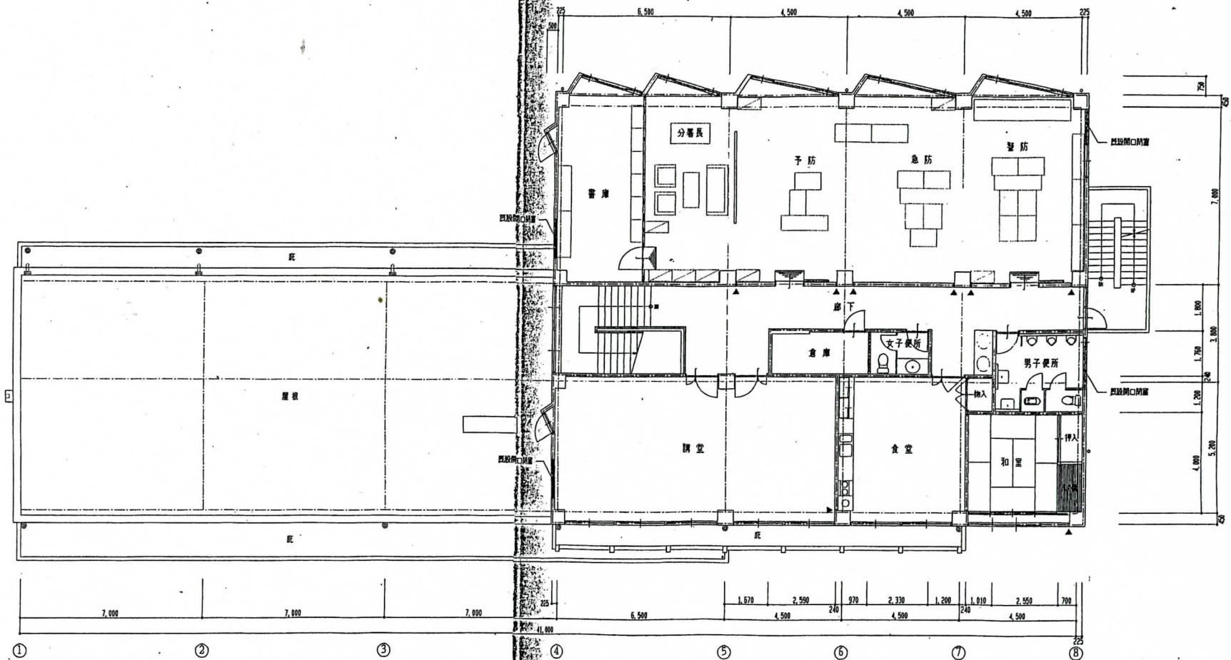
(改修) 2階平面図
