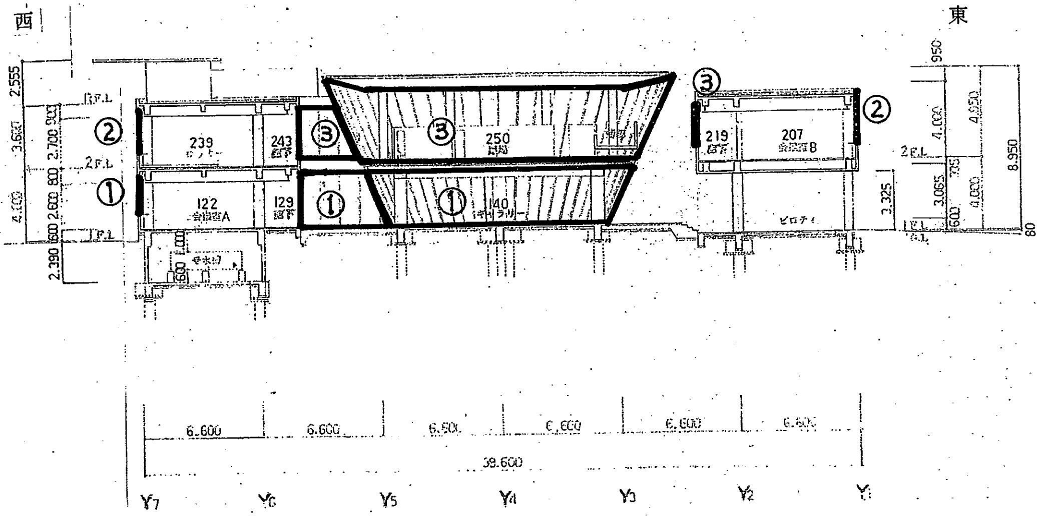
庵治支所立面図 (窓ガラス清掃) 中央広場より北の立面図
