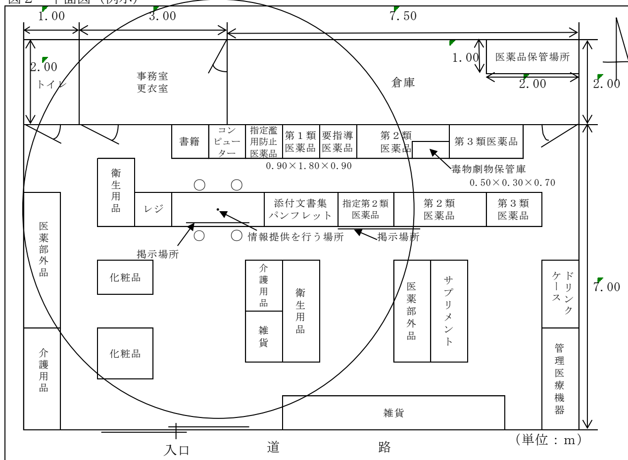
図2 平面図（例示）
