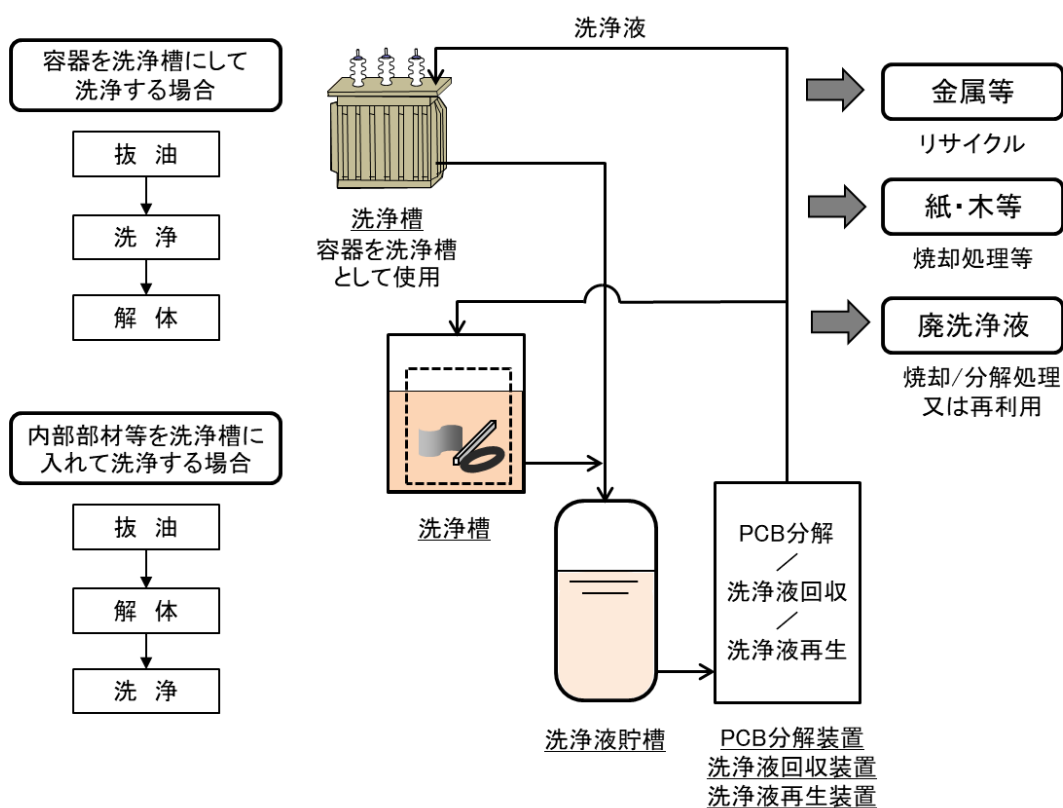
P C B に汚染された絶縁油を含む電気機器等の洗浄施設の例
