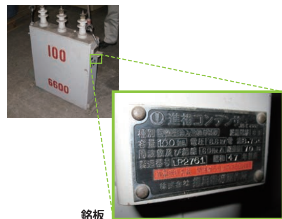
銘板
