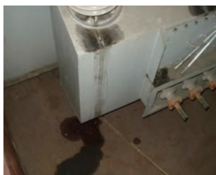
にじみ漏れの例（悪い例）
