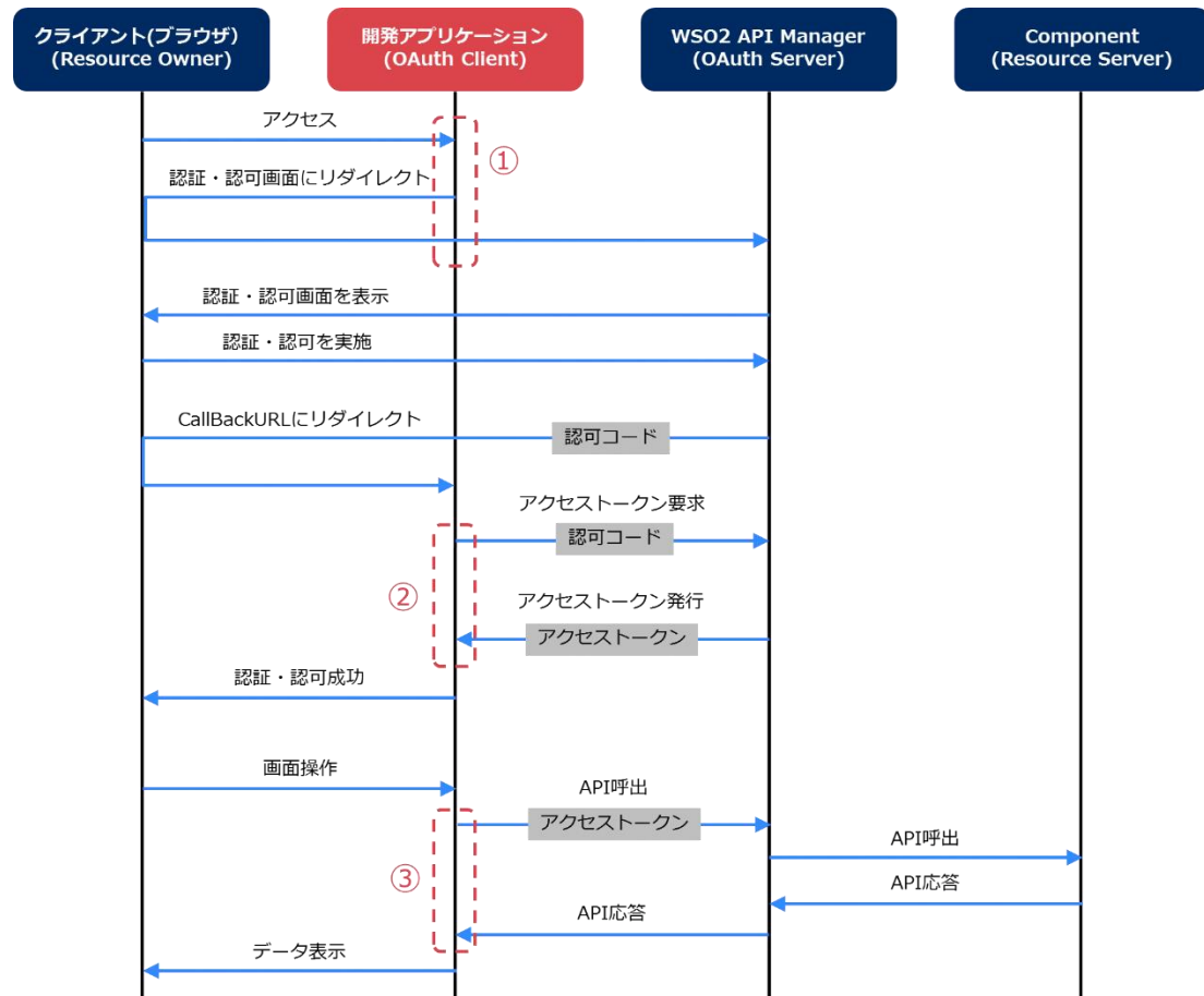
図 3-1 OAuth 2.0 認証のシーケンス(Authorization Code Grant)
