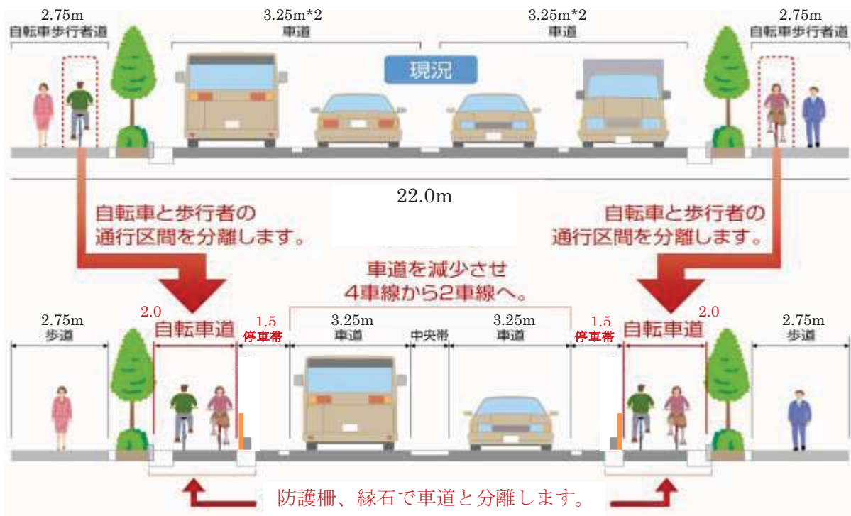
自転車道整備イメージ（五番町西宝線）
