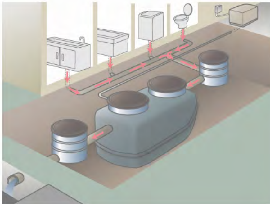
合併処理浄化槽
