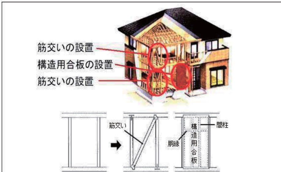
住宅耐震改修のイメージ
