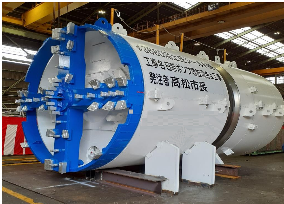
日新ポンプ場放流きよ工事用シールドマシン
