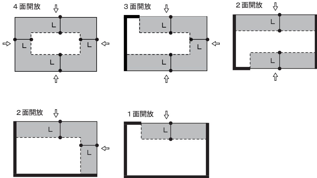
有効な吹きさらし部分(L:外気に面する5m未満の場所( ))の部分の例
