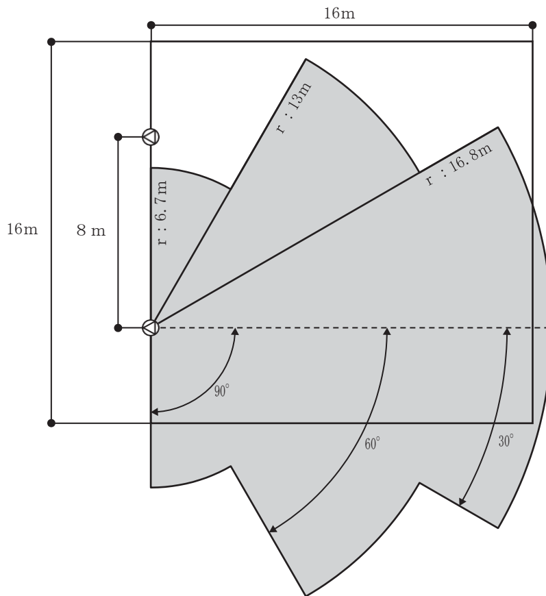
[側面図]
