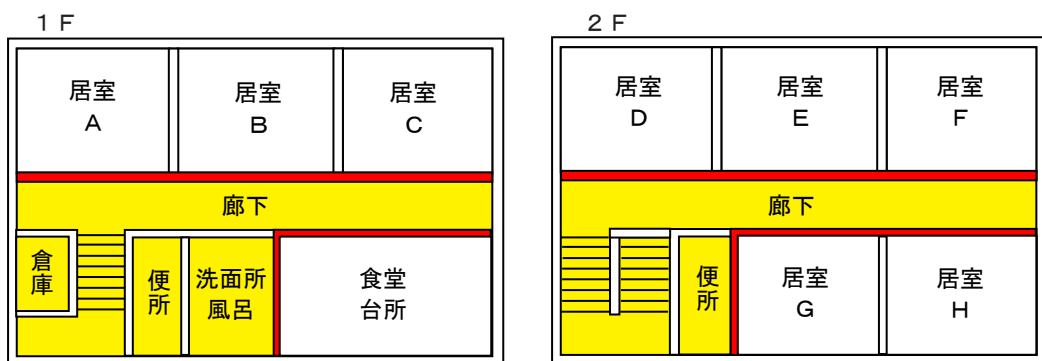
（2の階にわたって一の12条の2区画を設ける場合の例）
